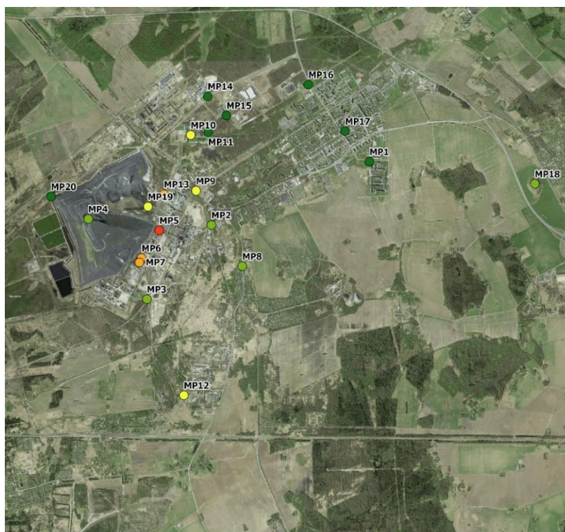
Joonis 48 Ksüleeni nädalakeskmine kontsentratsioon, 09.07 – 16.07.24
