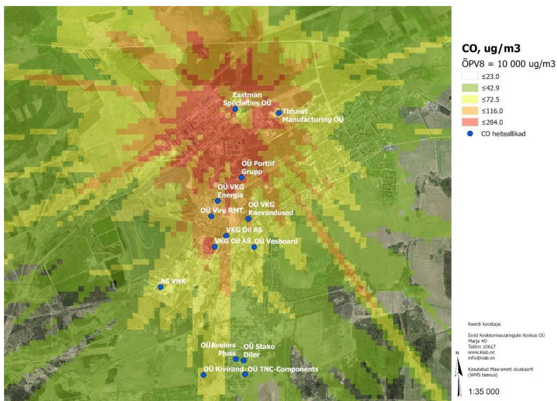
Joonis 21 CO 8 h maksimaalne kontsentratsioon KOTKAS 2023 a. andmete põhjal
