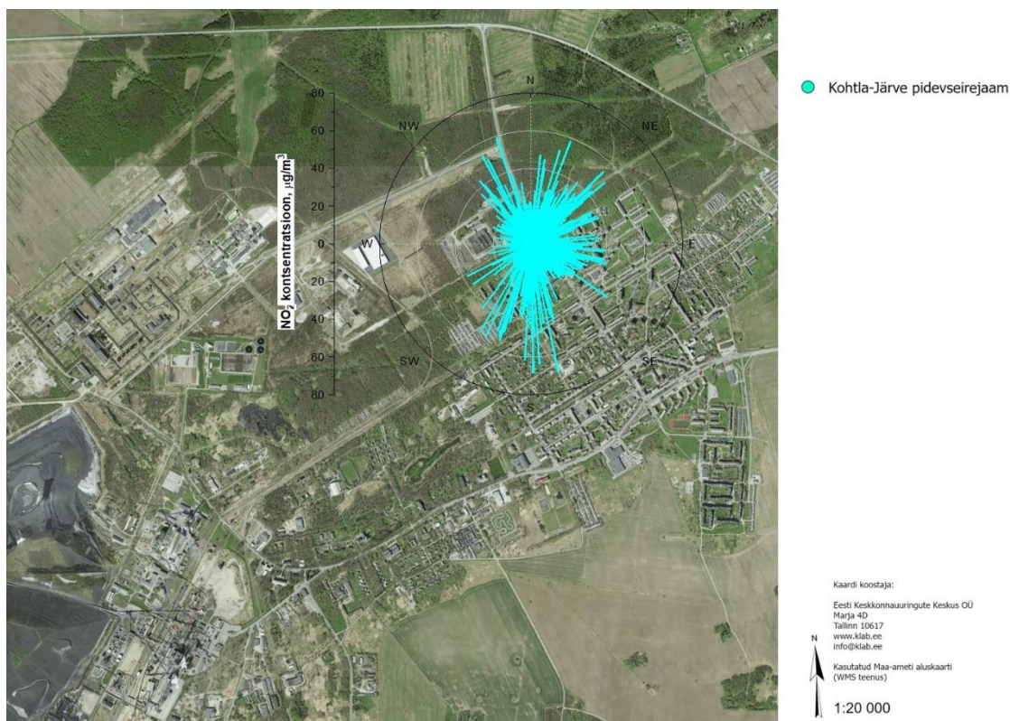
Joonis 123 NO 2 kontsentratsiooniroos, Kohtla-Järve seirejaam
