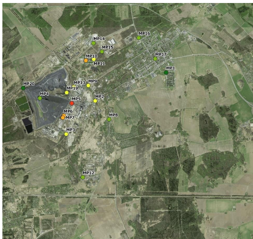
Joonis 49 Ksüleeni nädalakeskmine kontsentratsioon, 13.08 – 19.08.24
