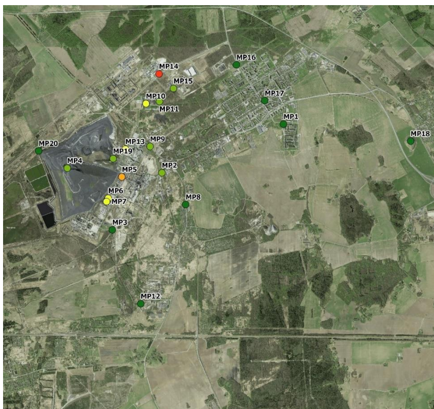
Joonis 56 Tolueeni nädalakeskmise kontsentratsioon, 09.07 – 16.07.24
