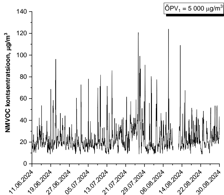
Joonis 81 NMVOC 1 h keskmine kontsentratsioon
