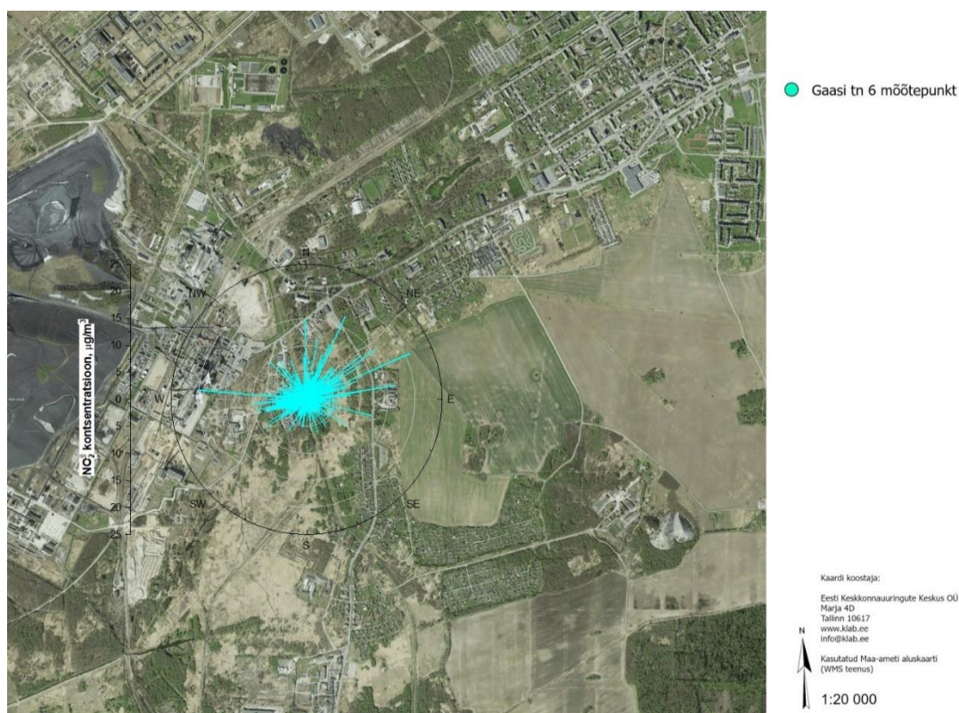
Joonis 94 NO 2 kontsentratsiooniroos, Mobair-2 mõõtepunkt
