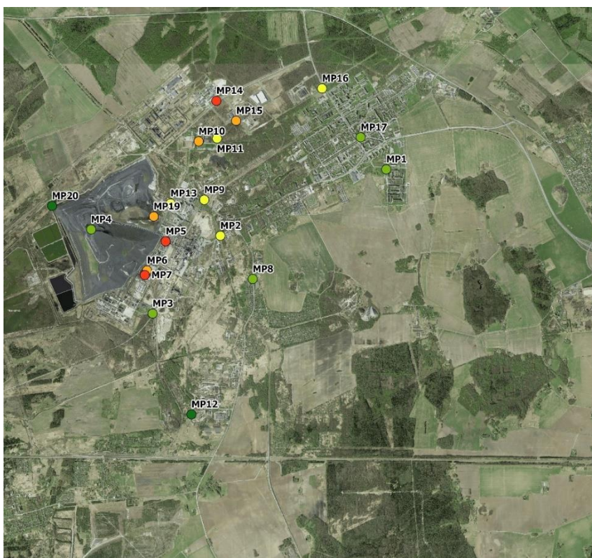
Joonis 57 Tolueeni nädalakeskmise kontsentratsioon, 13.08 – 19.08.24
