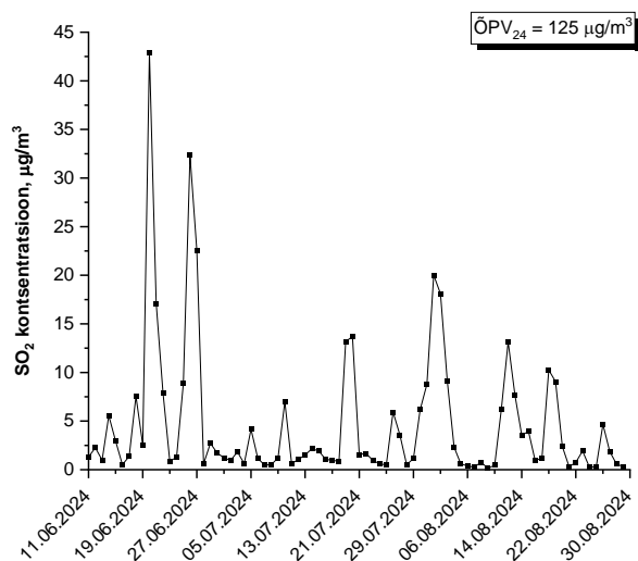
Joonis 89 SO2 24 h keskmine kontsentratsioon
