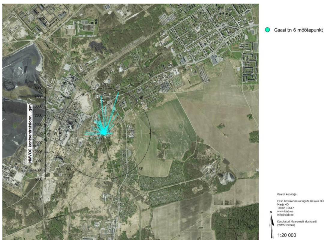
Joonis 107 NMVOC kontsentratsiooniroos, Mobair-2 mõõtepunkt
